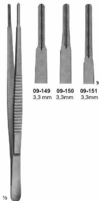
DE BAKEY 09-149 200 mm 09-150 240 mm 09-151 300 mm
